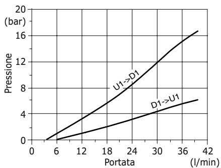
Diagramma perdite di carico VODL/SC 38 D1->U1 e U1->D1
